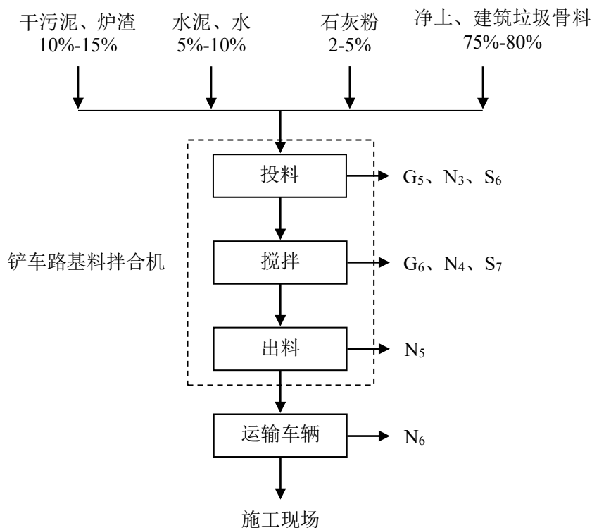
图2-4 污泥制路基商品灰土生产工艺流程及产污环节图
