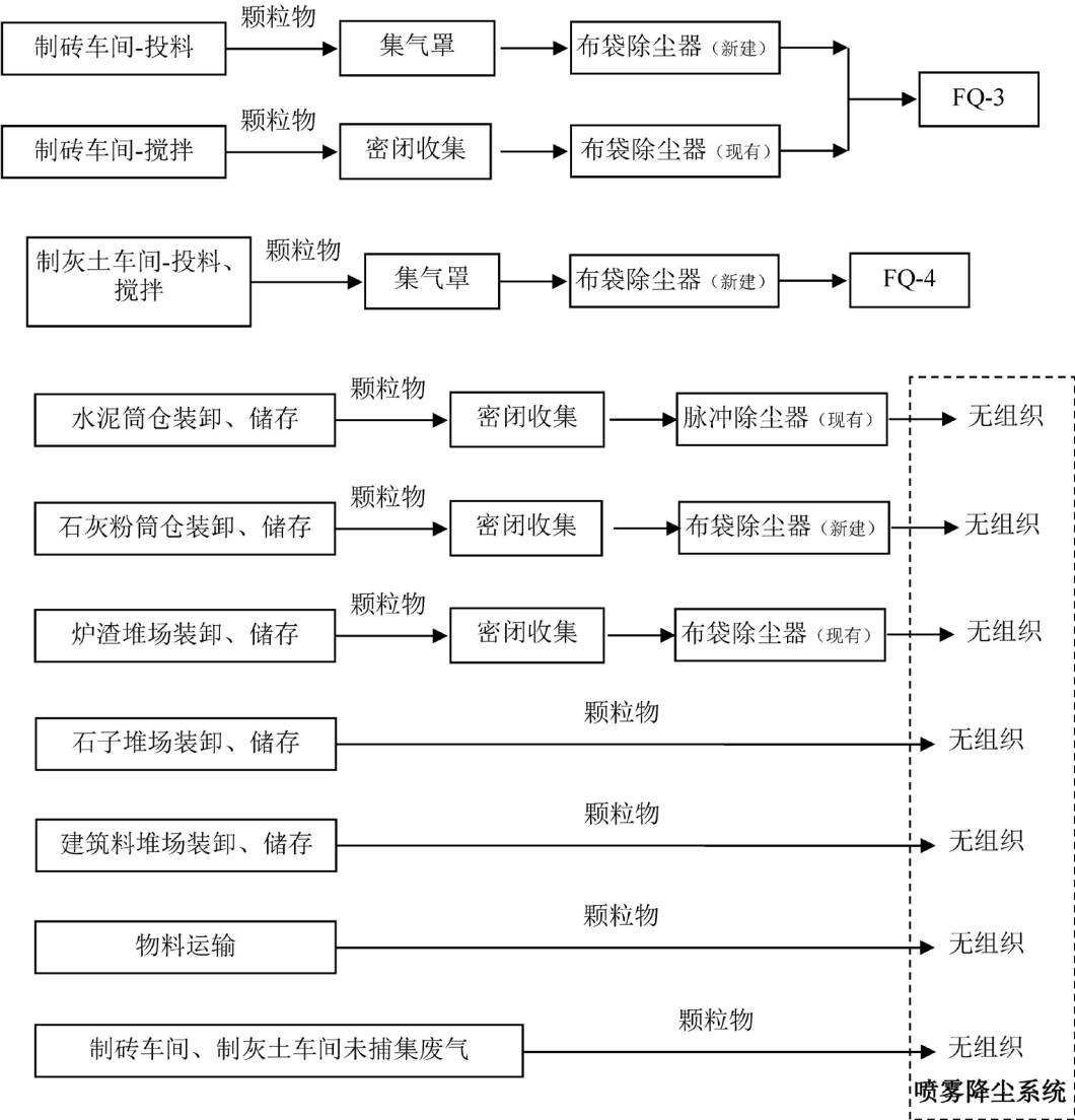
图4-1 本项目废气污染治理方案示意图
