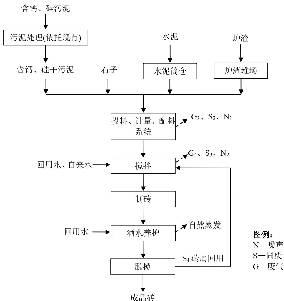
图2-3 污泥制混凝土实心砖生产工艺流程及产污环节图
