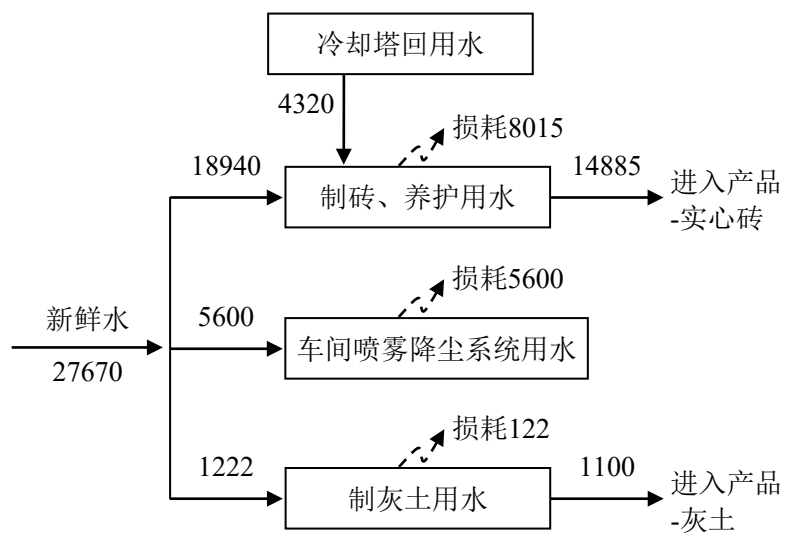
图2-1 本项目水量平衡图 （单位：吨/年）
