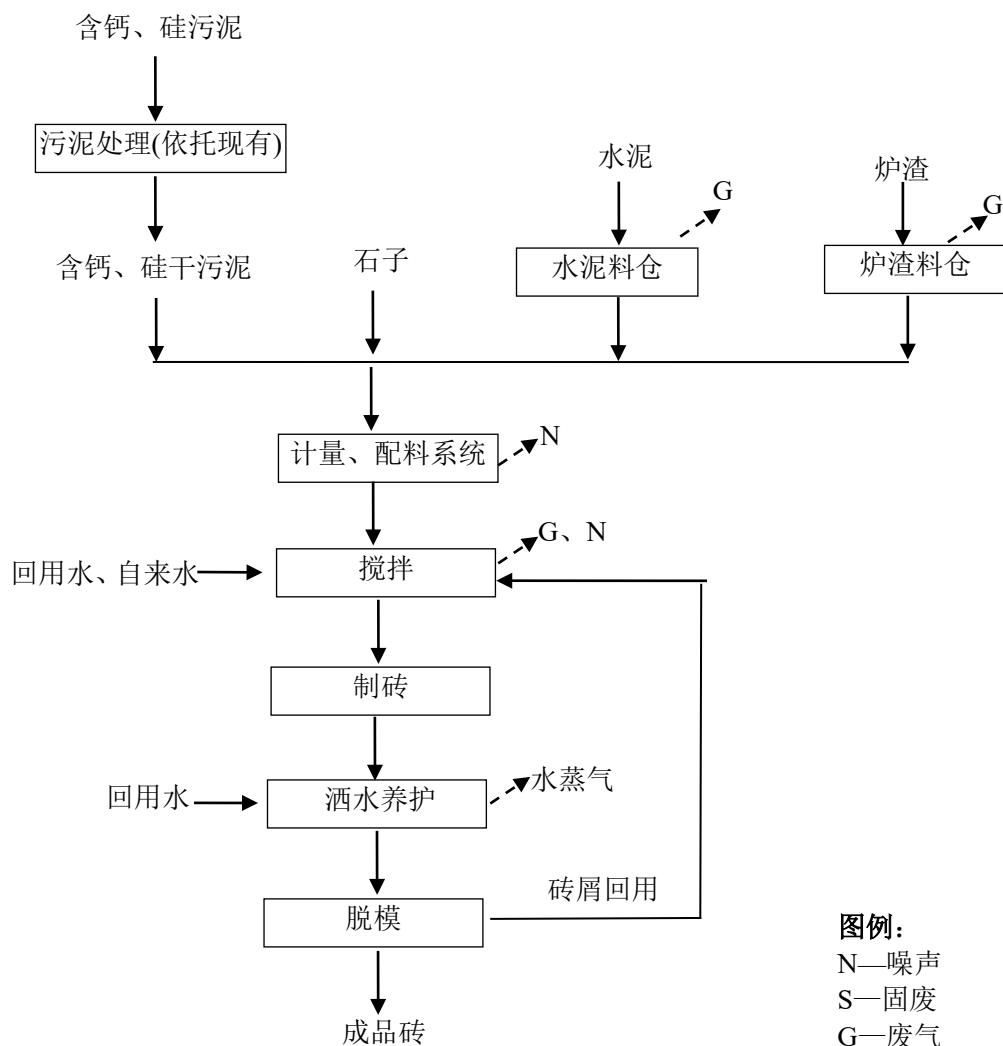
图2-7 制道板砖生产工艺流程及产污环节图
