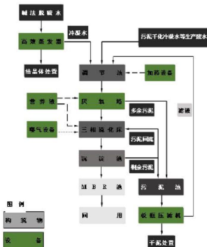
图2-9 污水处理工艺流程图
