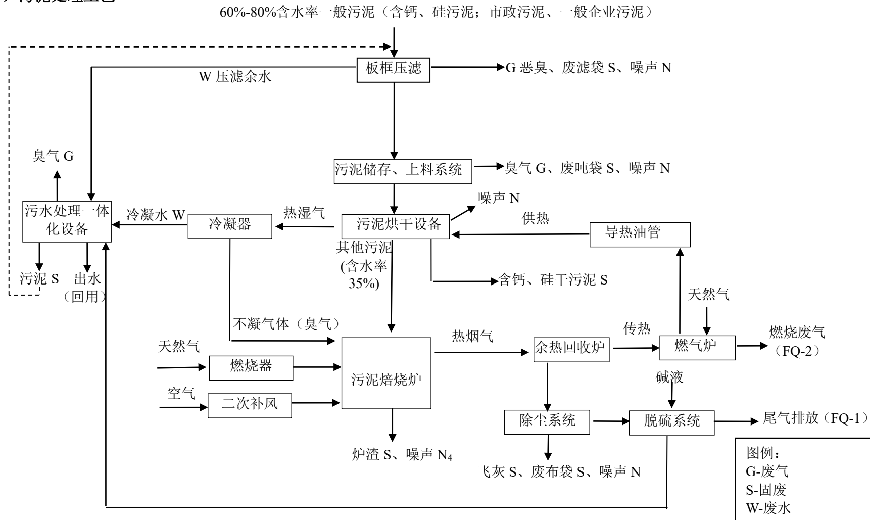
图2-5 污泥烘干、焙烧工艺流程及产污环节图
