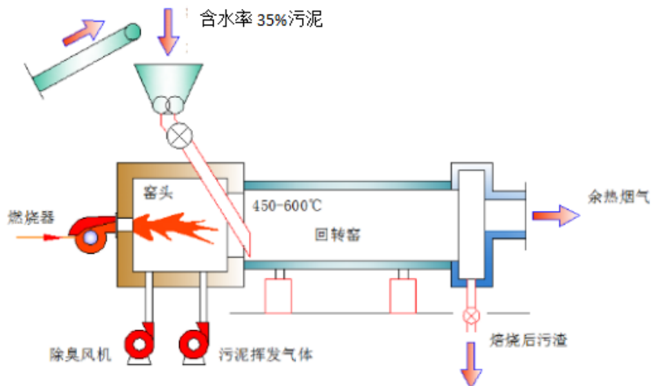
图2-6 焙烧炉结构示意图
